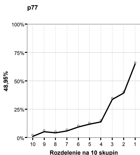
Obr. 11 Položka 77 – distribúcia úspešnosti a citlivosť
